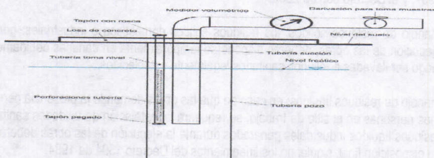
Figura 2. Instalación dispositivos de control al pozo
