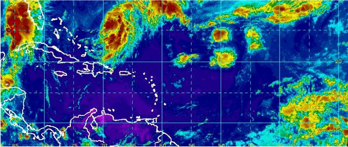
Imagen de satélite del canal infrarrojo Fecha: Septiembre 28 a las 10:15 a.m Hora Local Colombiana. Fuente. NOAA
