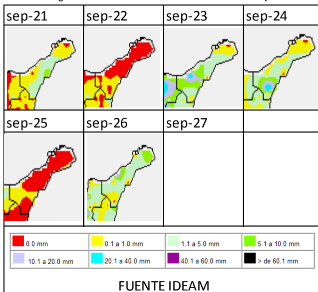
Figura 1 mosaico de lluvias diarias en La Guajira. Fuente IDEAM
