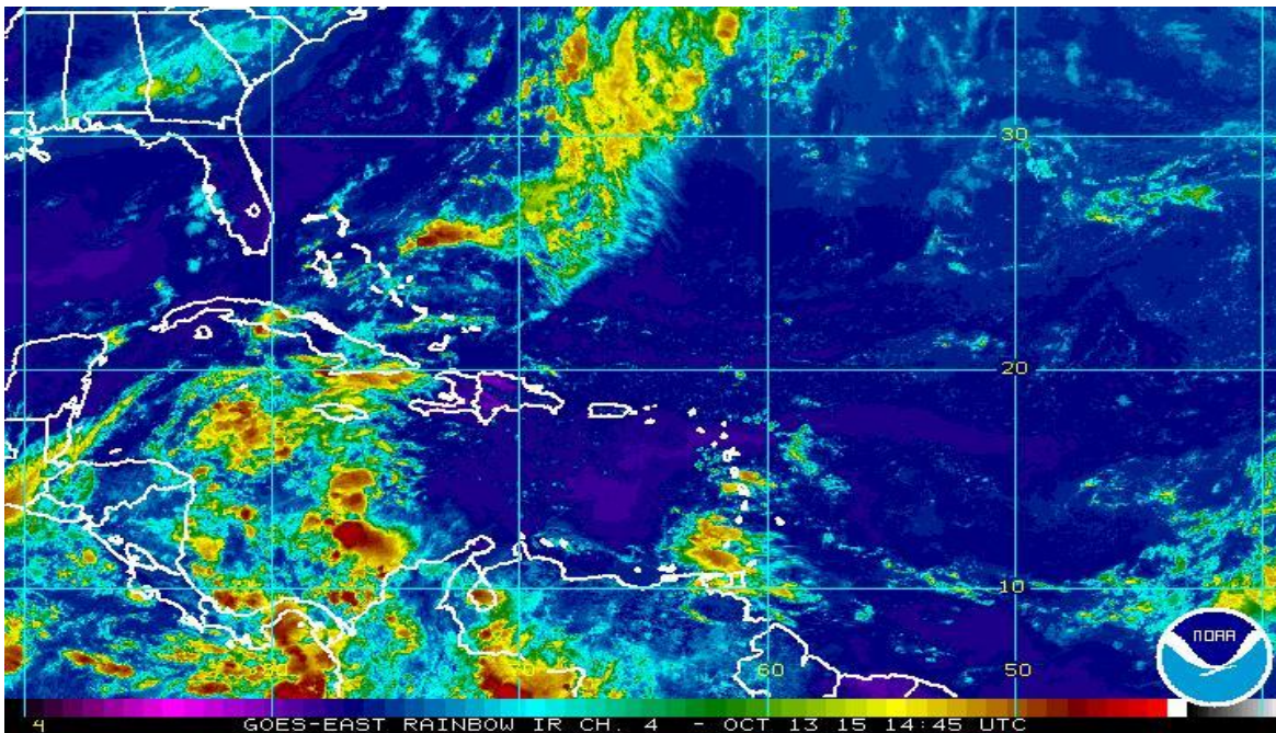
Imagen 2: Imagen satelital del canal infrarrojo Fecha: Octubre 13 a las 10:30 a.m Hora Local Colombiana. Fuente. NOAA.
